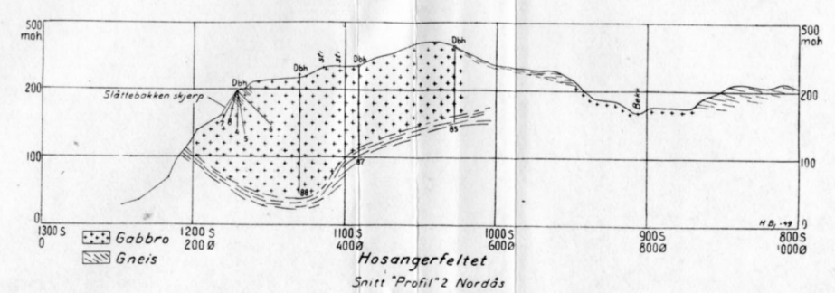
Profil gjennom gruvefeltet Hosanger. (Longitudinal Section)
