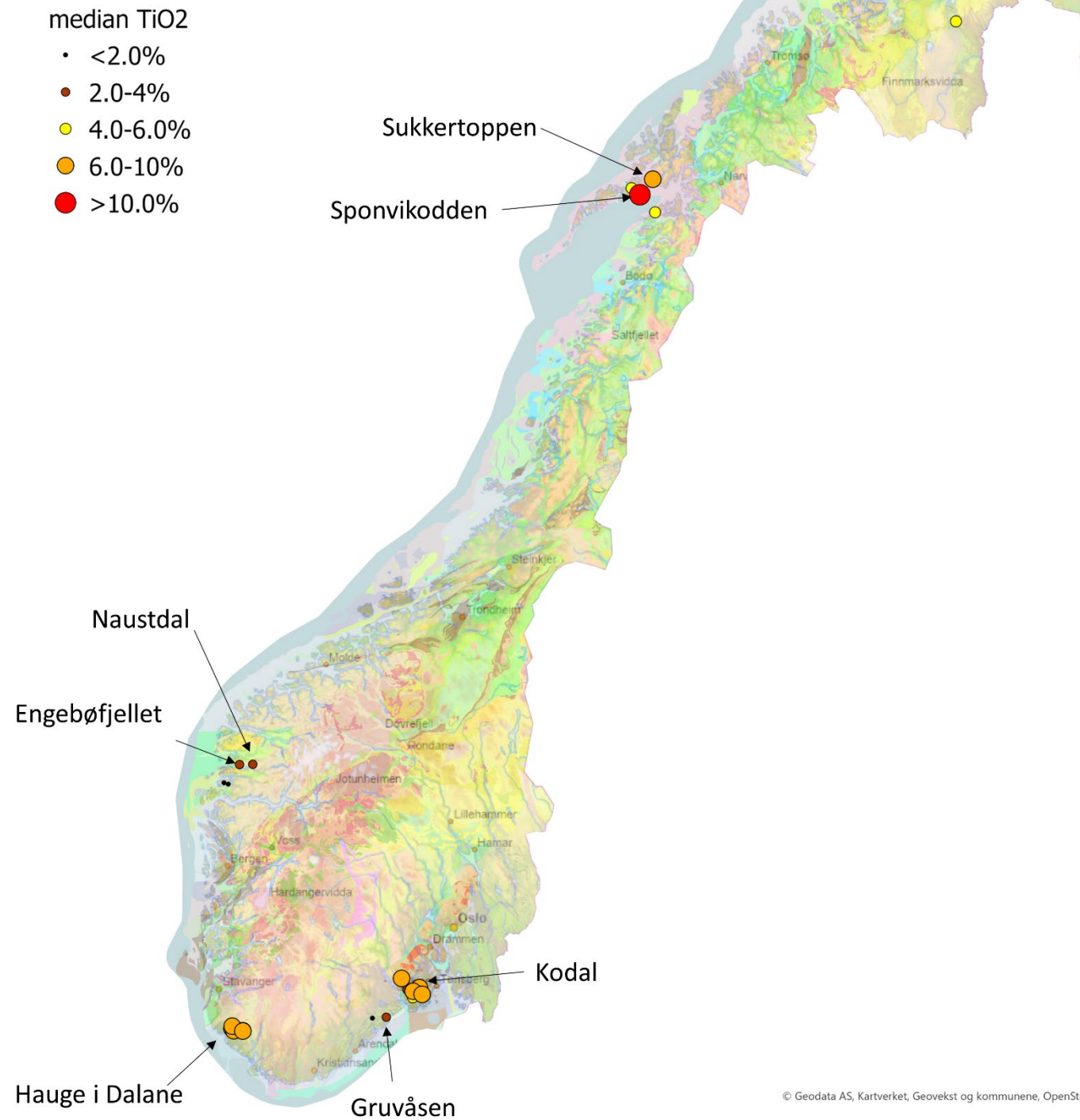
Figur 15 \text{TiO}_2 i ilmenitt og rutil registreringer (oksid-analyser).
