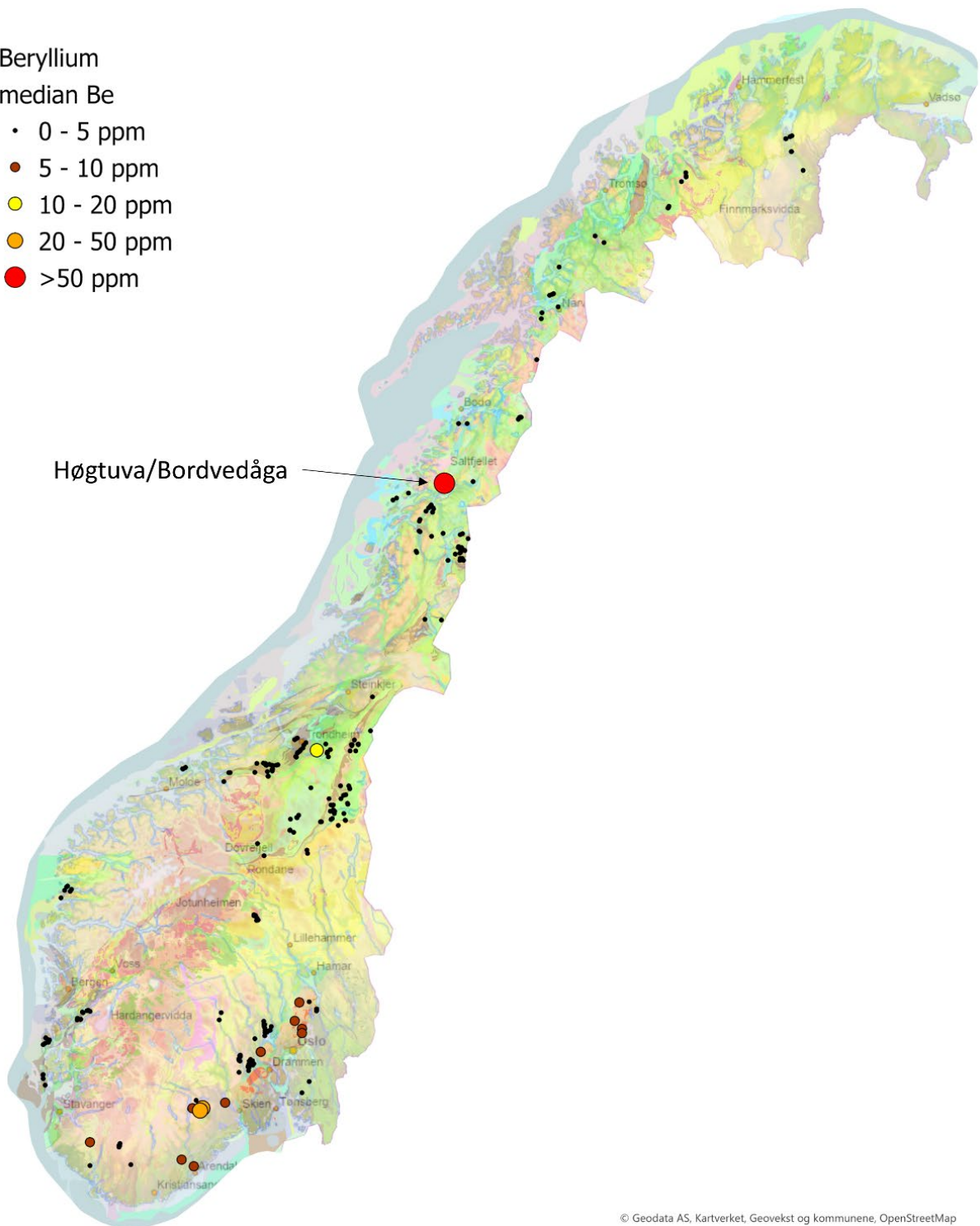
Figur 4: Beryllium-innhold i norske mineralregistreringer.
