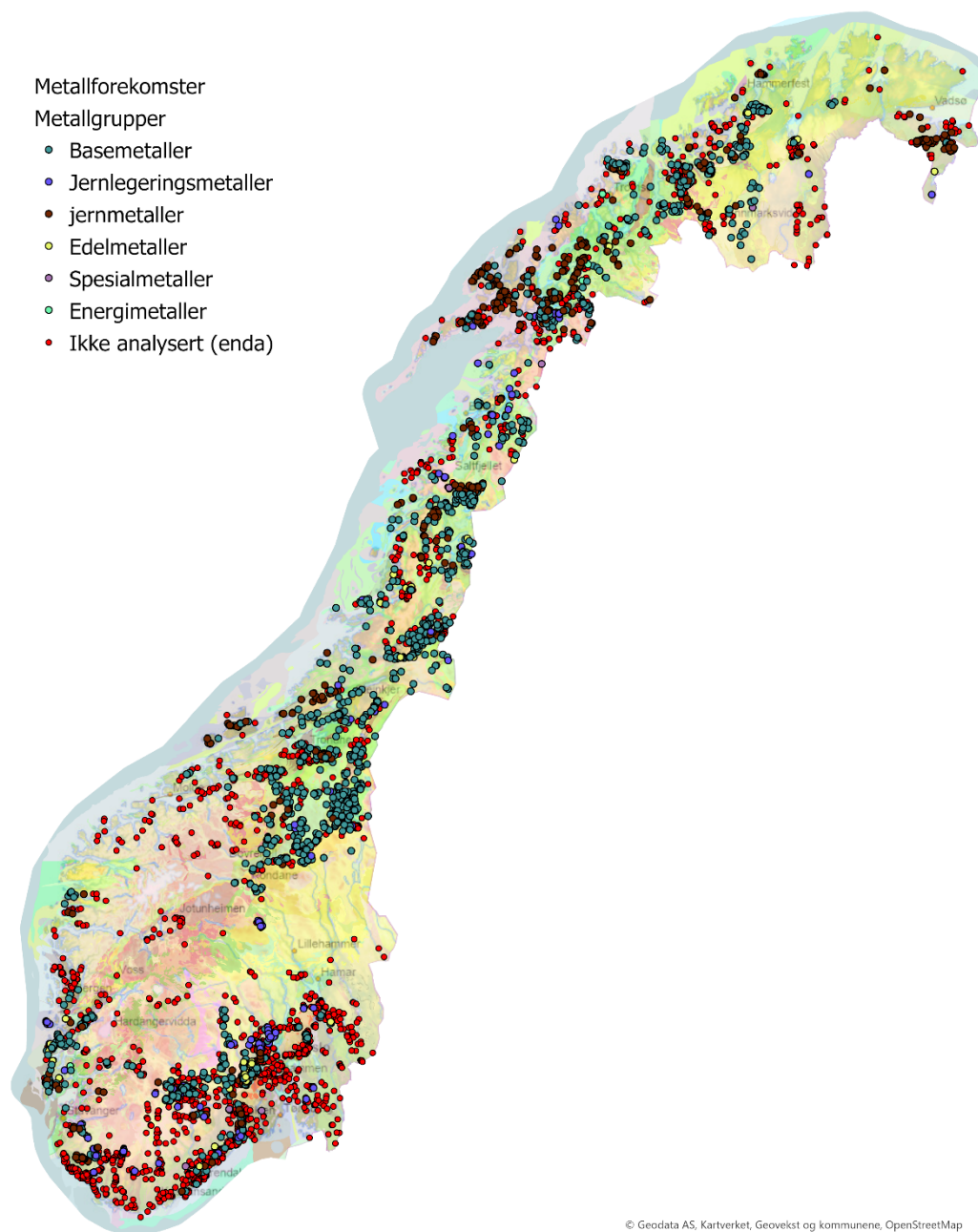
Figur 2: Forekomster og registreringer klassifisert etter metallgruppe. Symboler i rødt markerer registreringer som mangler analyser. De fleste av disse er heller ikke bekreftet. Vær oppmerksom på at punkttettheten også avspeiler kartleggingsgrad og kunnskapsnivå.
