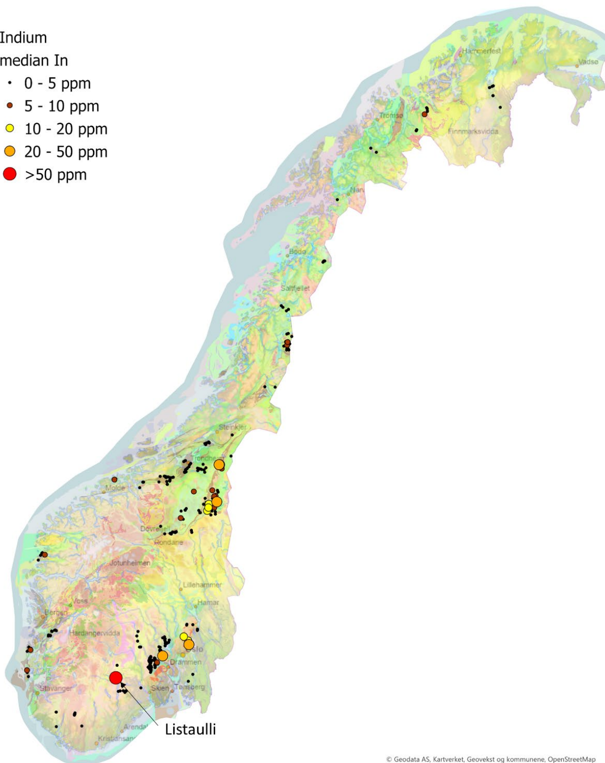
Figur 5: Indium-innhold i norske mineralregistreringer.
