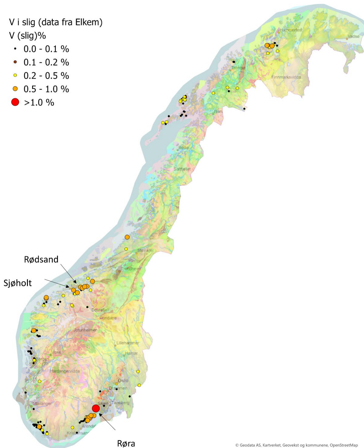
Figur 18: Innhold av vanadium i slig (magnetitkonsentrat).
