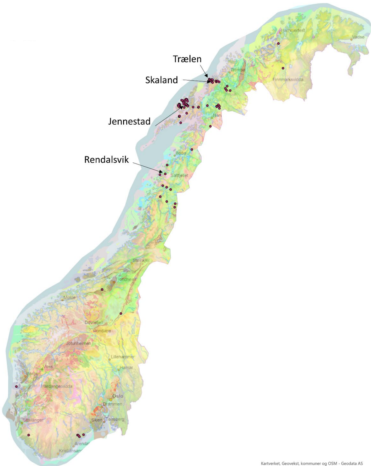
Figur 28: Norske grafitt-registreringer. Forekomster som er, eller har vært i drift, er navnsatt.
