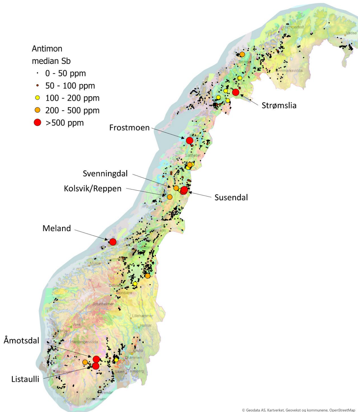
Figur 3: Antimon-innholdet i norske mineralregisteringer.
