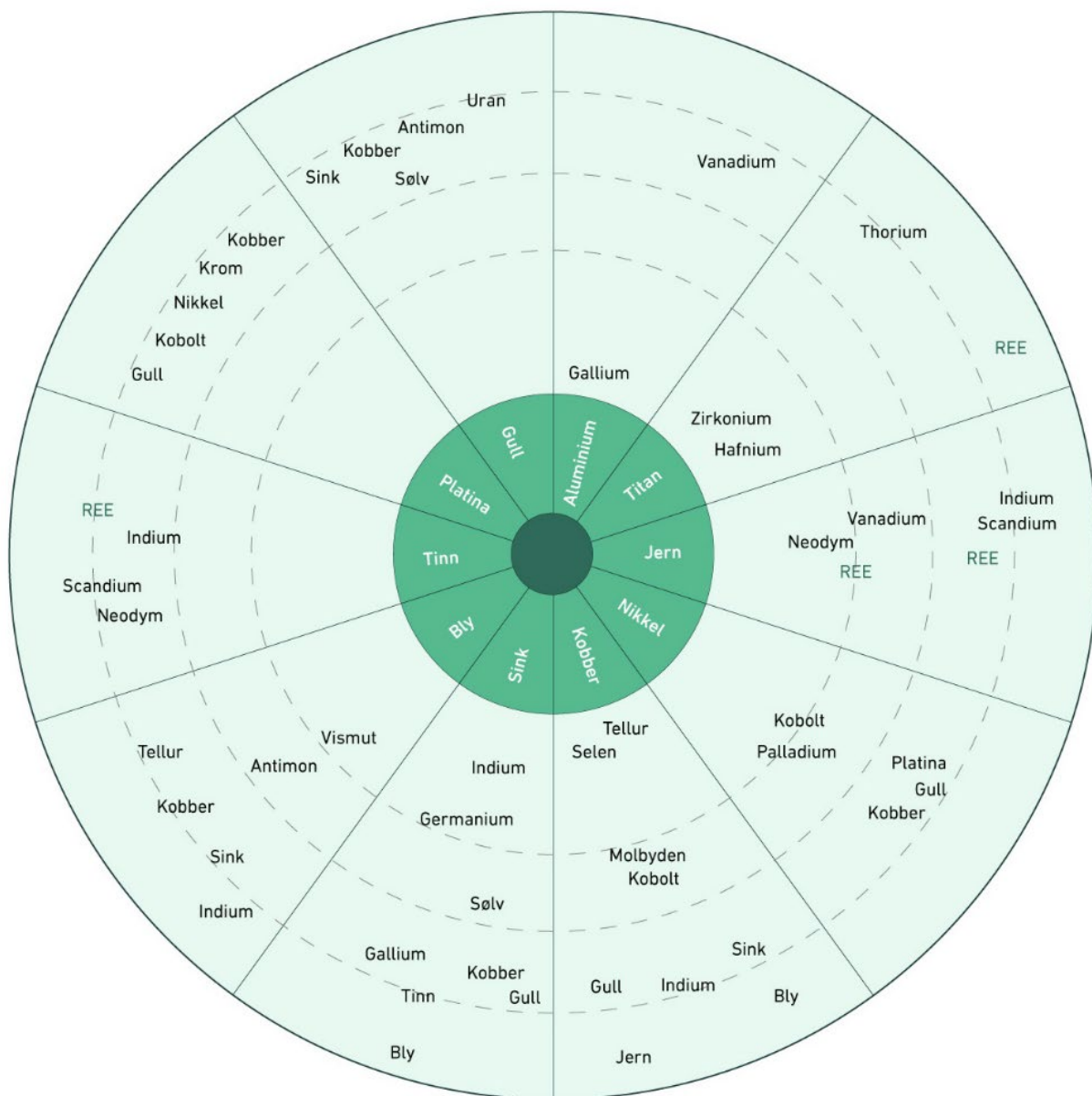
Figur 1: Hoved- og bimetaller, indre sirkel viser hovedmetallene mens assosierte bimetaller med avtagende grad av tilknytning ligger utover fra sentrum modifisert etter (Nassar et al., 2015). Figuren illustrerer fordelingen både for innhold og verdikomponenter.
