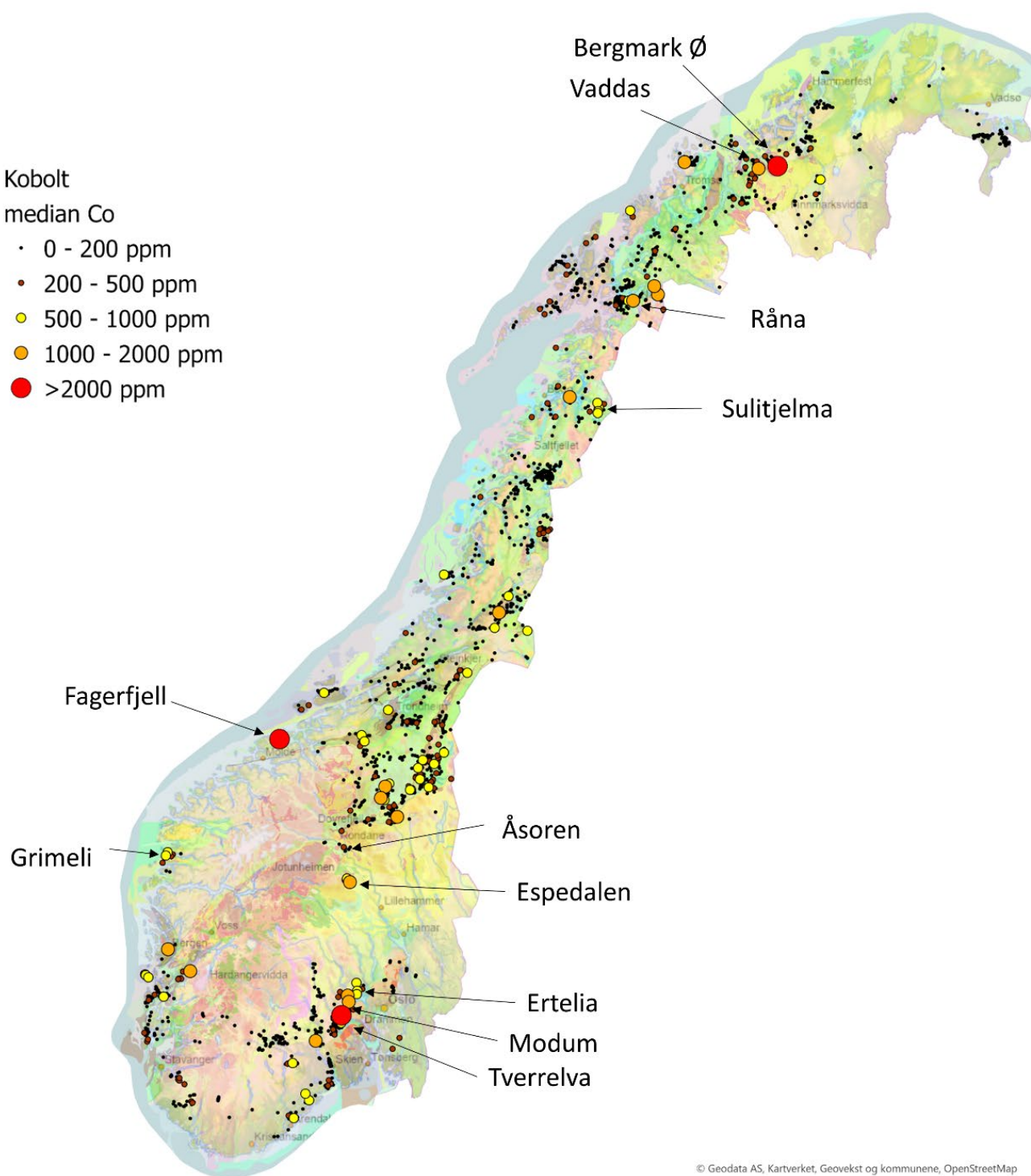
Figur 7: Kobolt-innhold i norske mineralregistreringer.
