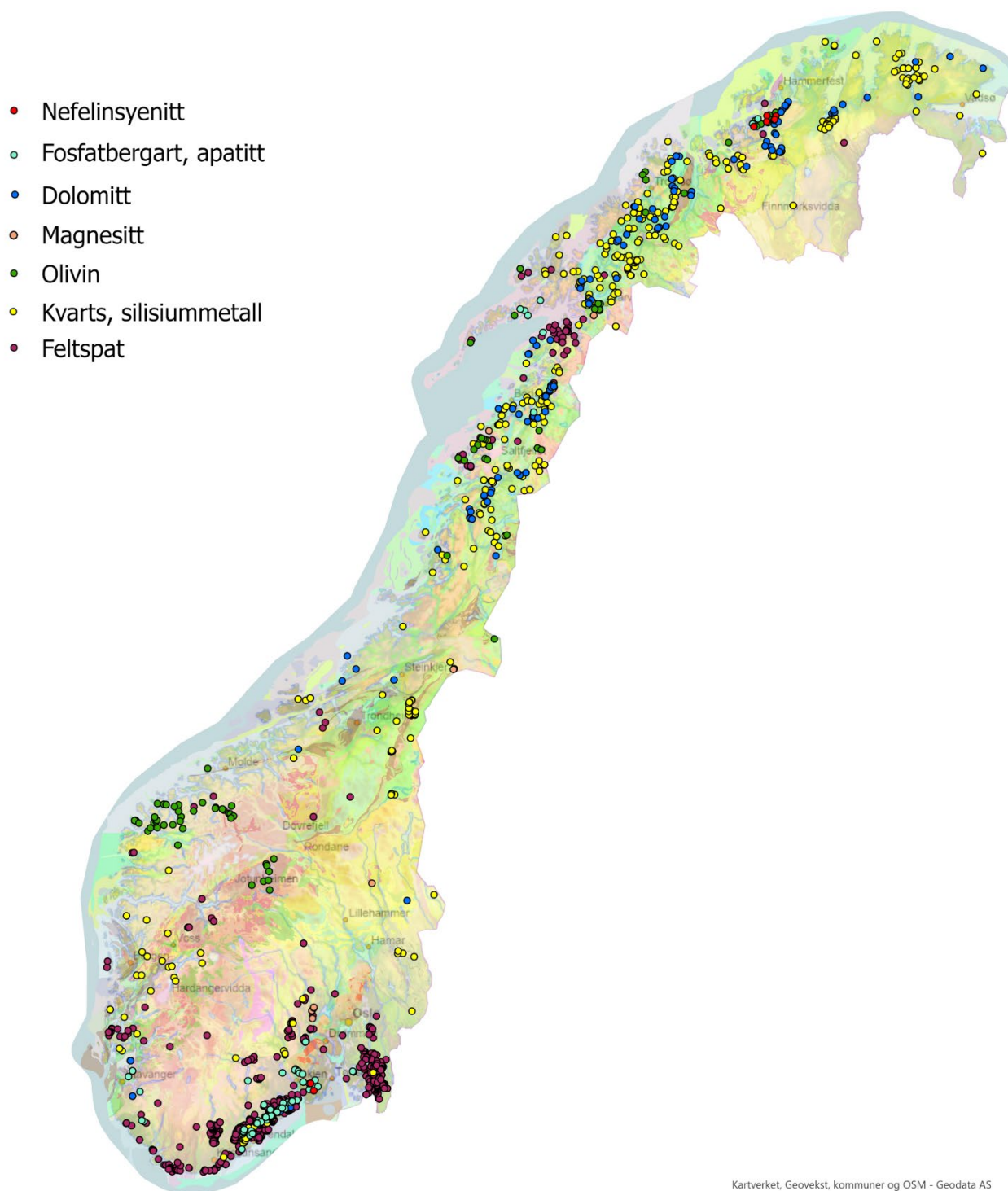
Figur 22: Forekomster og registreringer av kritiske og strategiske industrimineraler, inkludert industrimineraler som kan bli råstoff for kritiske raffinerte metaller.
