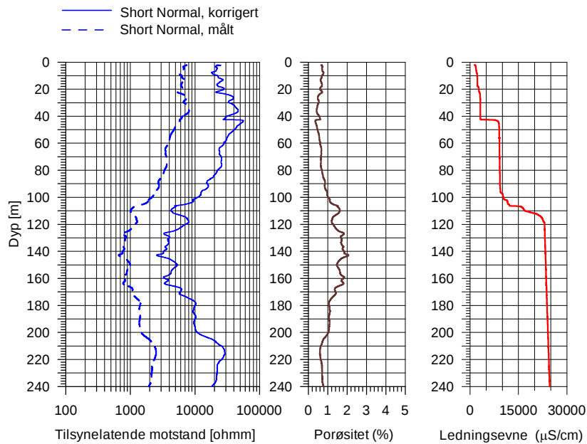
Figur 4. Eksempel på målt og korrigert resistivetslogg og beregnet porøsitet. Kurve til høyre viser variasjonen i vannets elektriske ledningsevne (inngår i beregningene).
