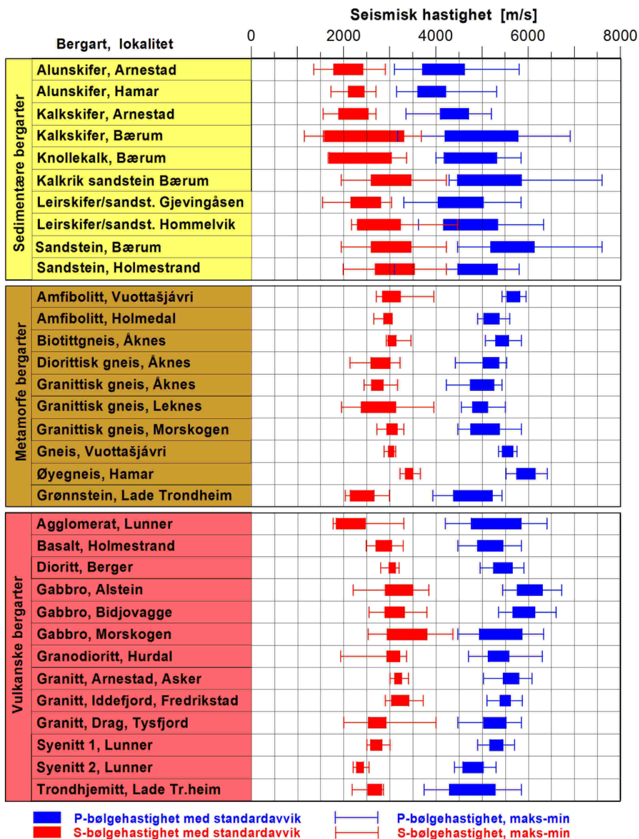
Figur 14: Seismiske hastigheter i ikke oppsprukne norske bergarter.
