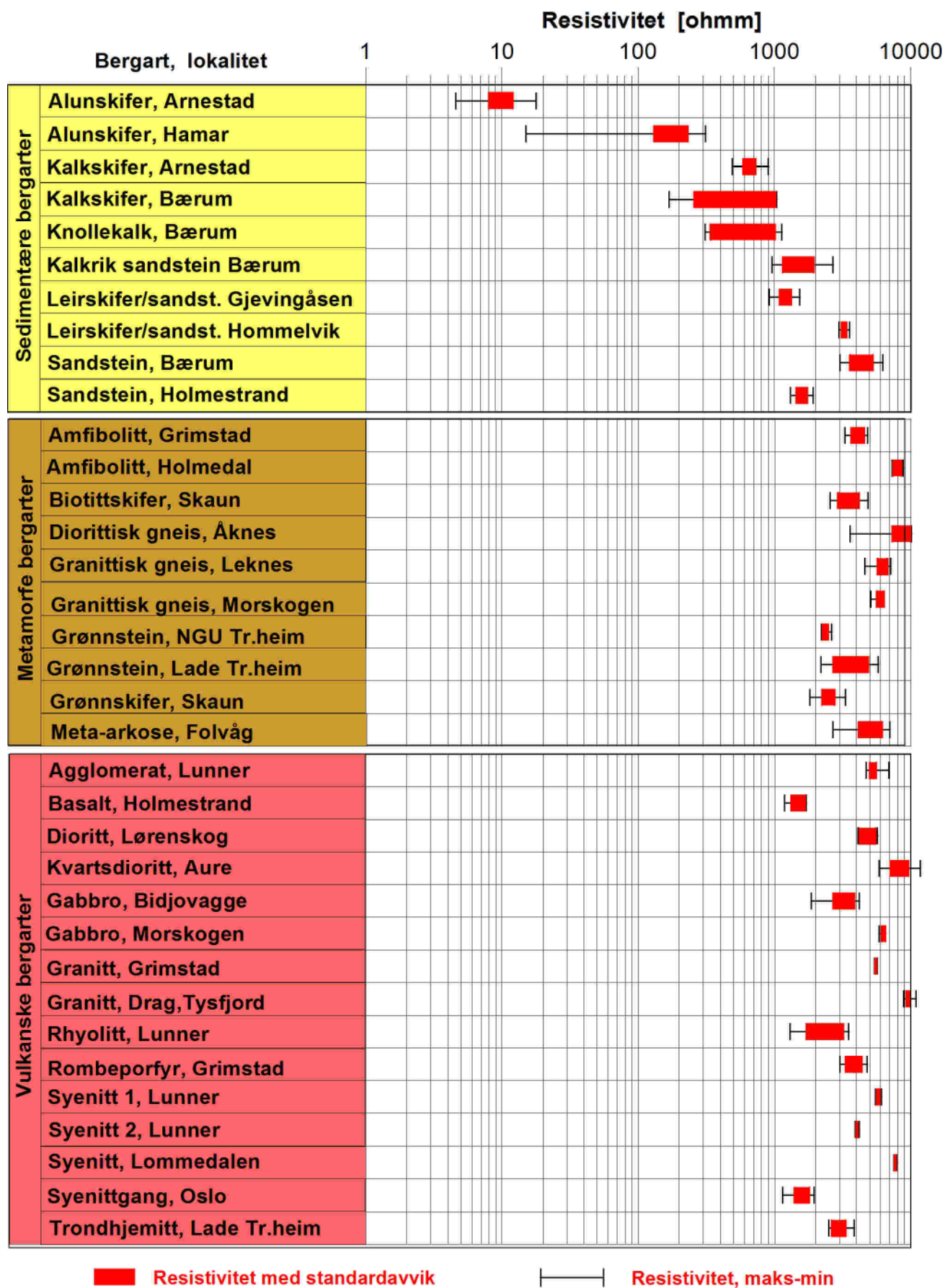
Figur 13: Resistivitet i ikke oppsprukne norske bergarter.
