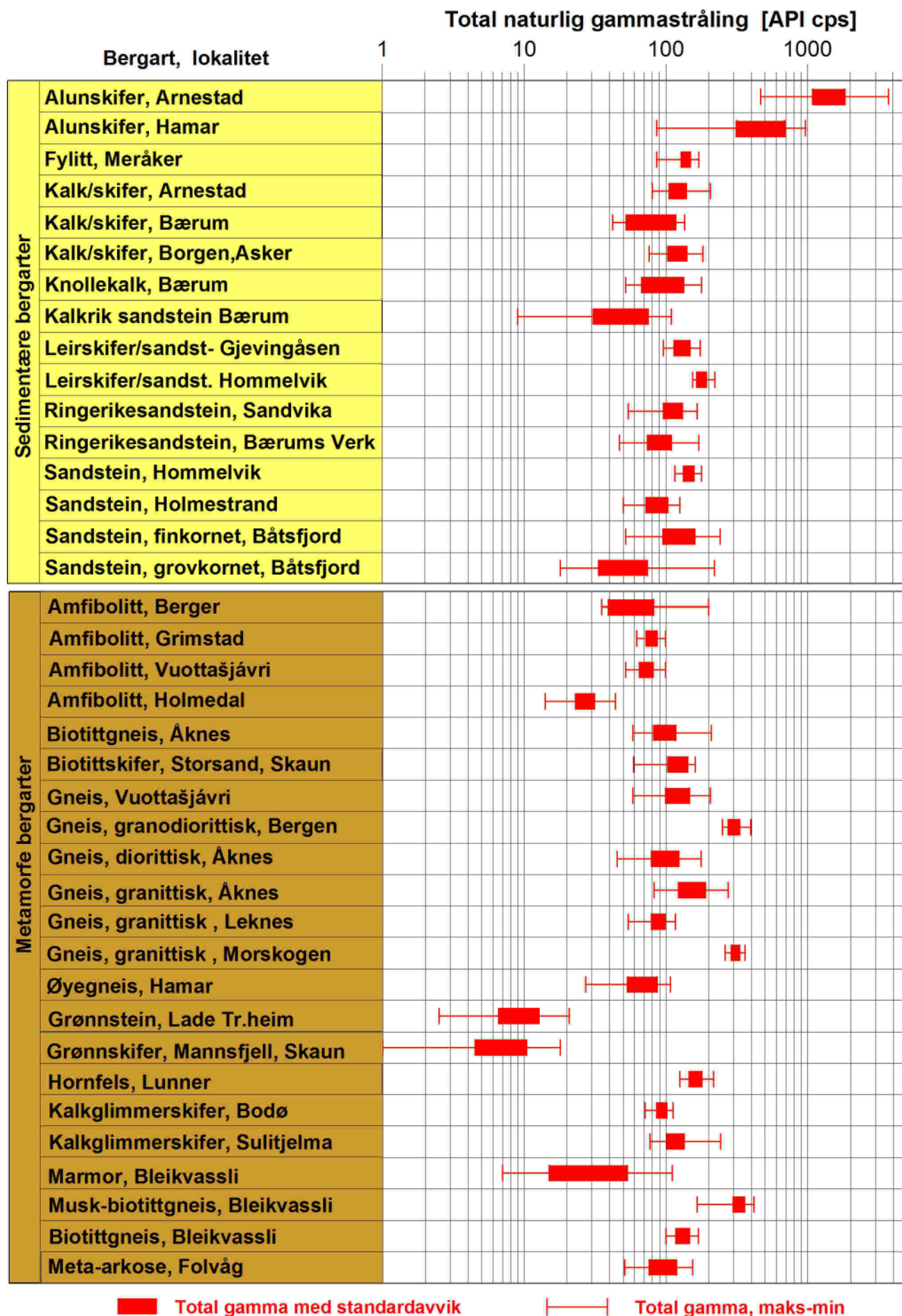
Figur 15: Naturlig gammastråling i norske bergarter.
