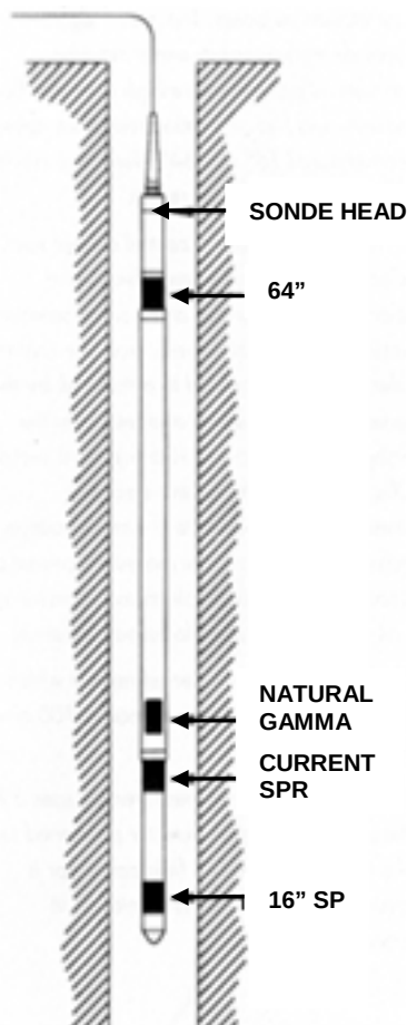
Figur 3. Resistivitets-sonde.
