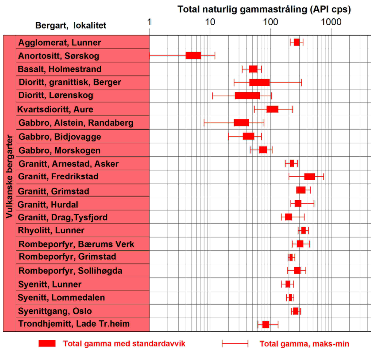
Figur 15(forts.): Naturlig gammastråling i norske bergarter.
