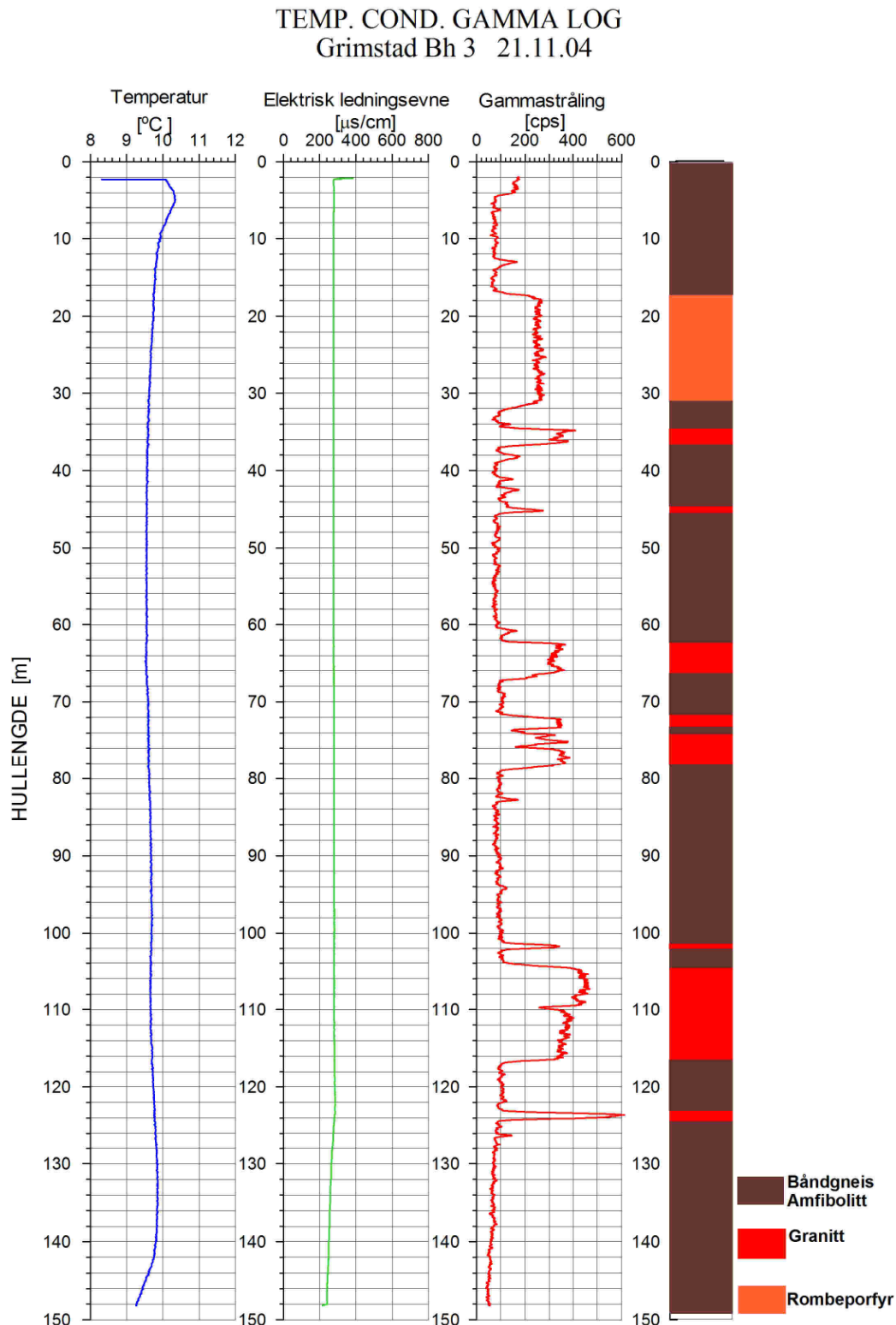
Figur 12. Bh 3 Grimstad. Temperatur, elektrisk ledningsevne i vann og naturlig gamma. Geologisk logg er basert på opptak med optisk televiwer.
