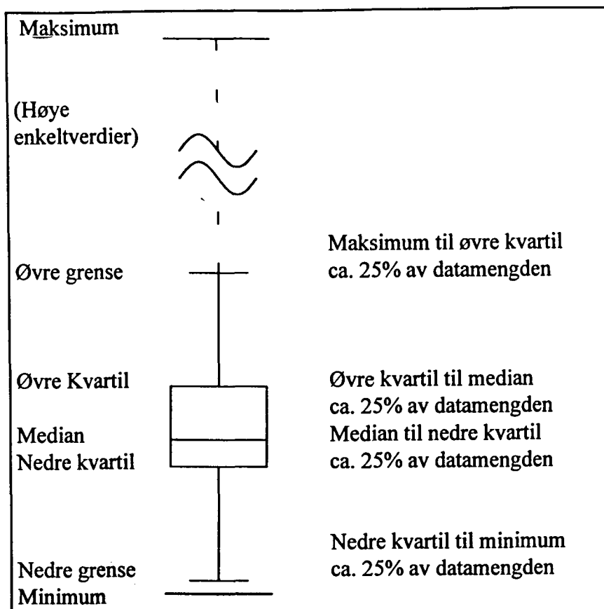
Figur 3: Grafisk forklaring av boksploTT
