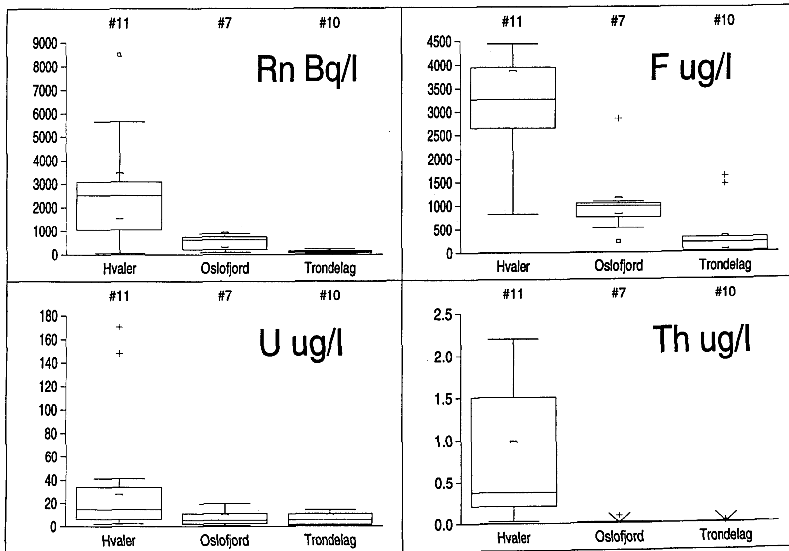
Figur 1: Utvalgte resultater fra tidligere undersøkelser av radon (Rn), fluorid (F), uran (U) og thorium (Th) i borebrønner i fjell.
