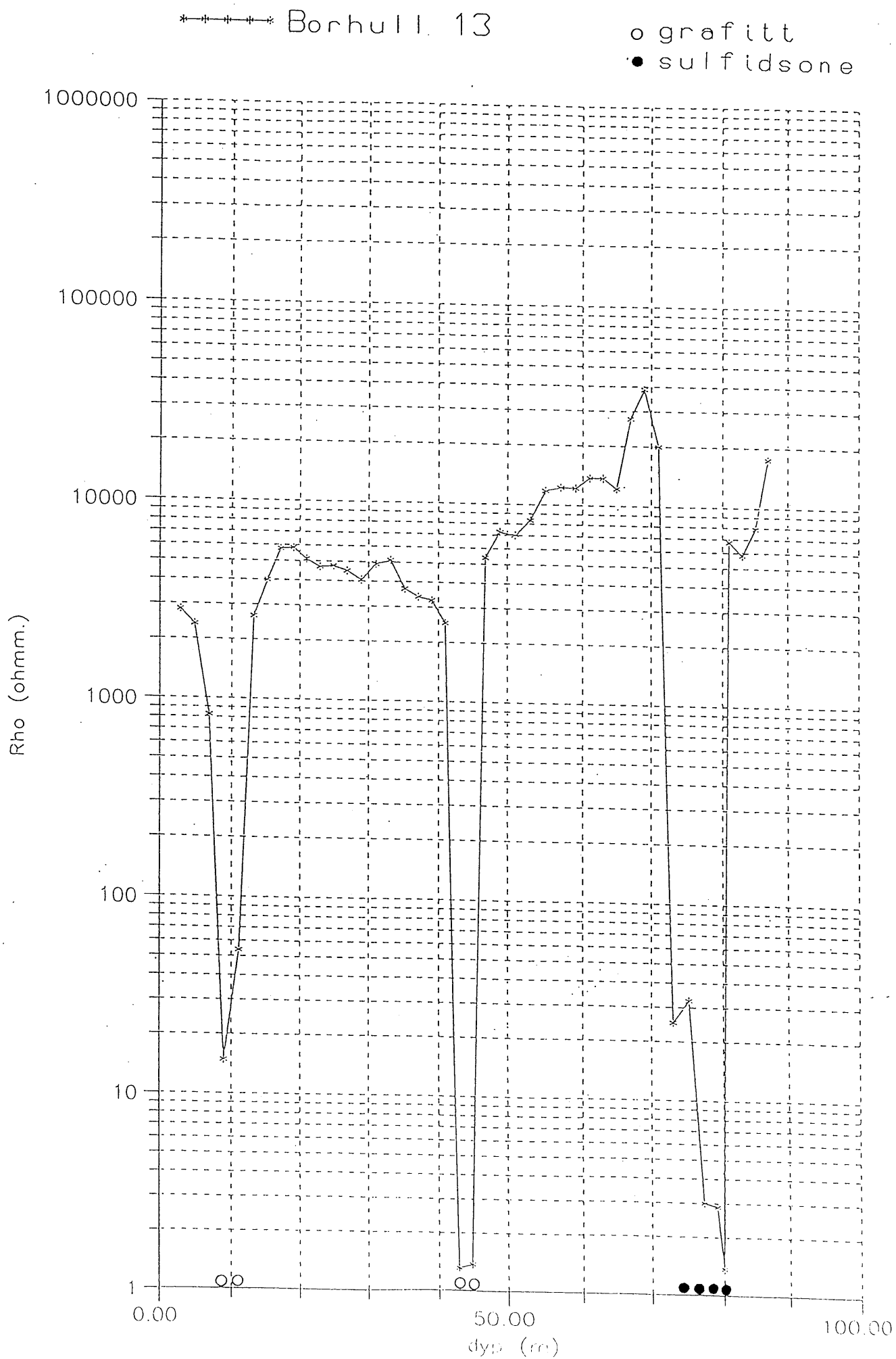
Figur 7. Ledningsevne-målinger borhull 13.
