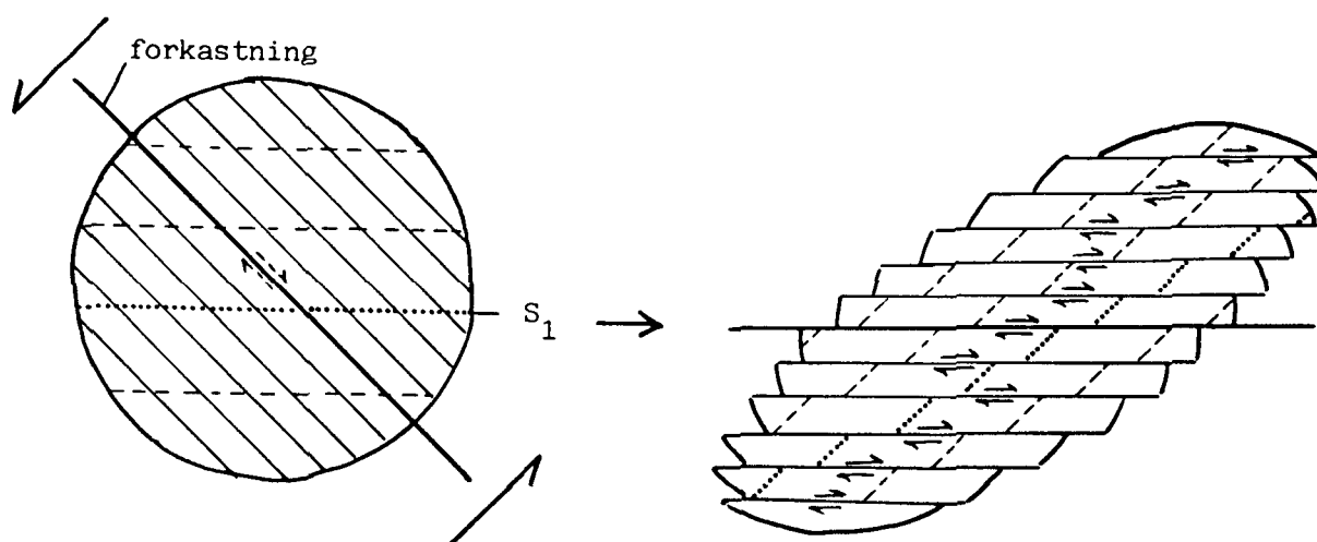
Fig. 5. Modell for homogen deformasjon ved rotasjon og forskyvning av stive plater. \Gamma = 1.0 , X/Z \approx 3 .
