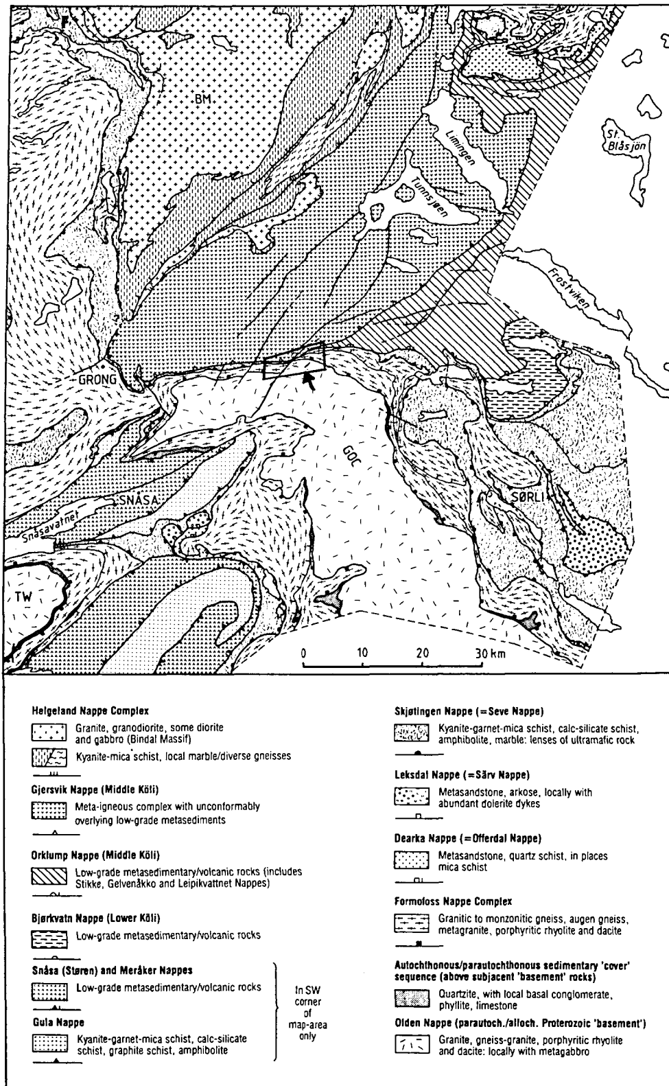
Fig.1: Tektonostratigrafisk kart (fra Roberts 1989) som viser den regionale plasseringen av det undersøkte område. GOC = Grong-Oldenkulminasjonen.
