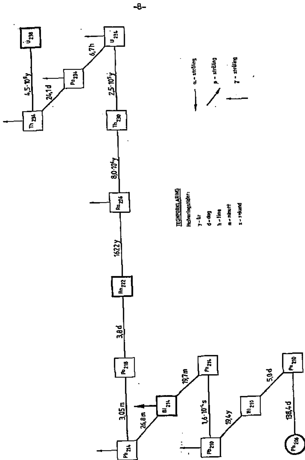
Fig. 1. Forenklet spaltningssække for uran 238, som er den mest vanlige uranisotop i naturen.
