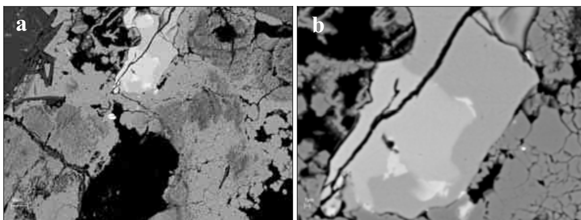
Figur 10 (a) SEM bse-bilde som viser relikv av (ikke omvandlet) sinkblende (grå) innesluttet i goethitt (varierende mørkere grå, omdannet fra magnetkis). (b) Detalj fra foregående bilde som viser 'normal' sinkblende (middels grå) og In-rik sinkblende (lysgrå). De hvite områdene er bismutinitt og matilditt.
