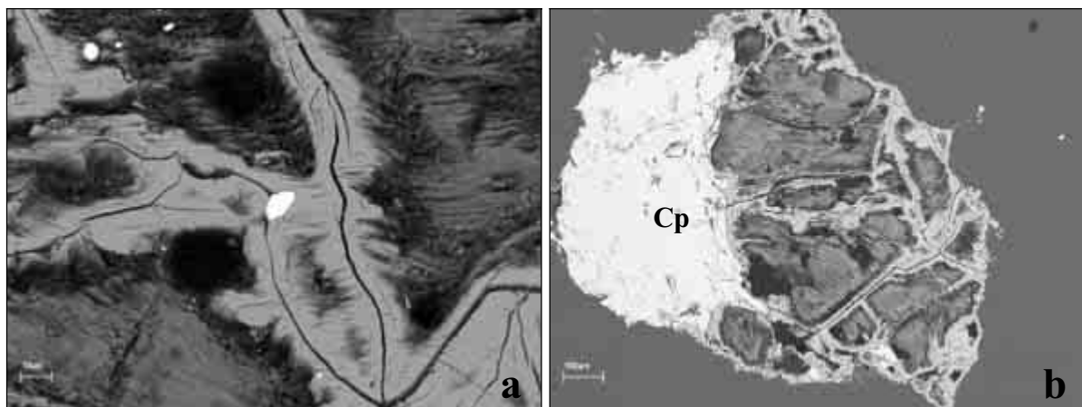
Figur 8: SEM bse-bilder som viser progressiv oksidasjon av magnetkis (a, b). Kobberkisen (Cp) er ikke påvirket av denne omvandlingsprosessen.
