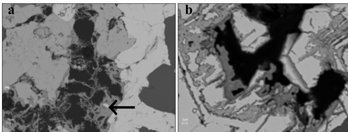
Figur 9: SEM bse-bilder som viser omvandling av svovelkis. (a) Randen av store svovelkiskorn (lys grå) er omvandlet til goethitt (grå, vist med pil). Sorte områder er hulrom. (b) Detaljbilde som viser oppløsning og total nedbrytning av svovelkis.
