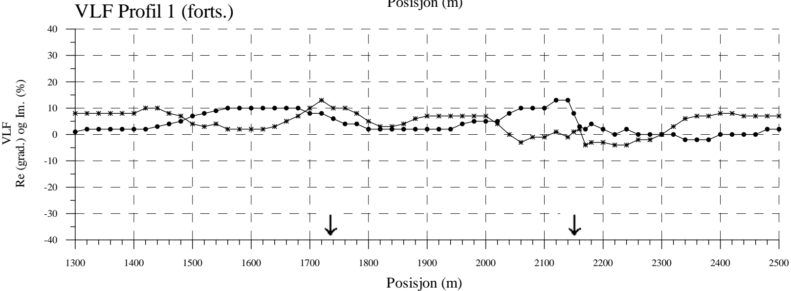
Figur 3. VLF profil 1
