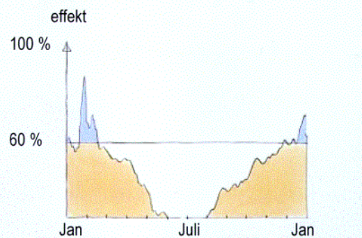
Figur 6. Fordeling av oppvarmingsbehov for en bolig gjennom året (Oslo Energi Enøk, 2002).
