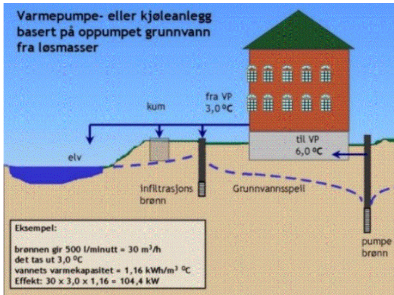
Figur 13. Eksempel på varmepumpe- eller kjøleanlegg som bruker opp-pumpet grunnvann fra løsmasser som energikilde. Varmevexlet grunnvann blir enten infiltrert i en nærliggende brønn, grøft, basseng, eller pumpet til et vassdrag.
