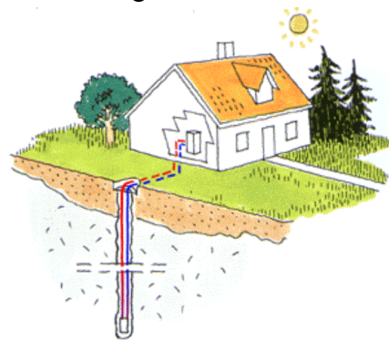
Figur 7. Prinsippkisse av grunnvarme fra borehull i fjell (lukket system) (Normann Energiteknikk, 2002).
