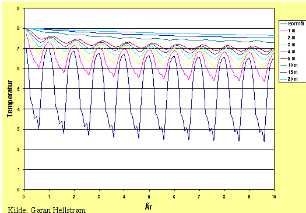
Kilde: Gøran Hellstrøm Figur 11. Temperaturutvikling i og omkring en energibrønn i fjell med lukket kollektor over en periode på 10 år. Den blå kurven representerer temperaturen i selve borehullet, mens de andre kurvene måler temperaturforholdene i radiell avstand fra brønnen (Hellstrøm, 2001).
