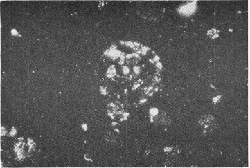
Fig. 3. Mikrofoto av rundt olivinkorn (chondrer) i Pollen-meteoritten (100 x). Photomicrograph showing olivinichondrite in the Pollen meteorite (100 x).
