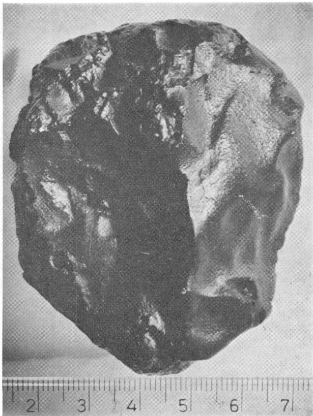
Fig. 2. Pollen-meteorittens bakside som viser piezoglypter.
