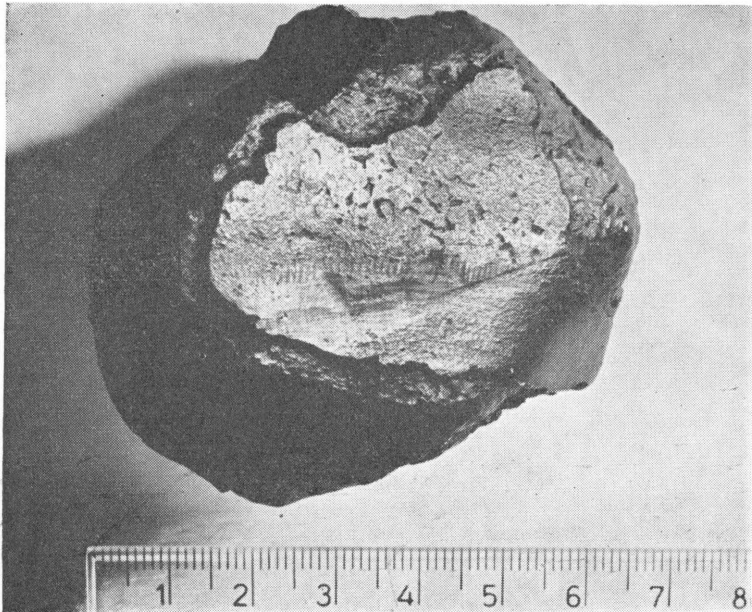
Fig. 1. Pollen-meteorittens frontalside som viser den 1 mm tykke smelteskorpen med kontraksjonsriss.
